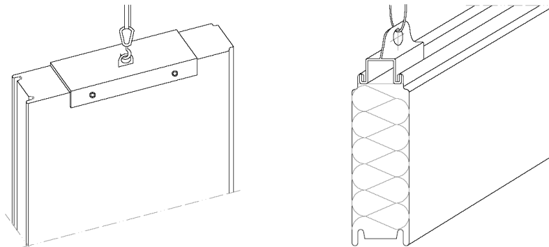
Рис.5. Схема механического захвата со сквозным сверлением панели (при вертикальном монтаже) Рис.6. Схема механического захвата, устанавливаемого в замок панели (при горизонтальном монтаже)
