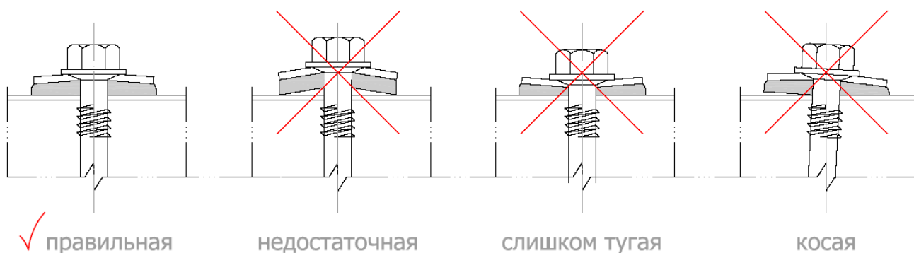
Рис.8. Посадка шурупов
