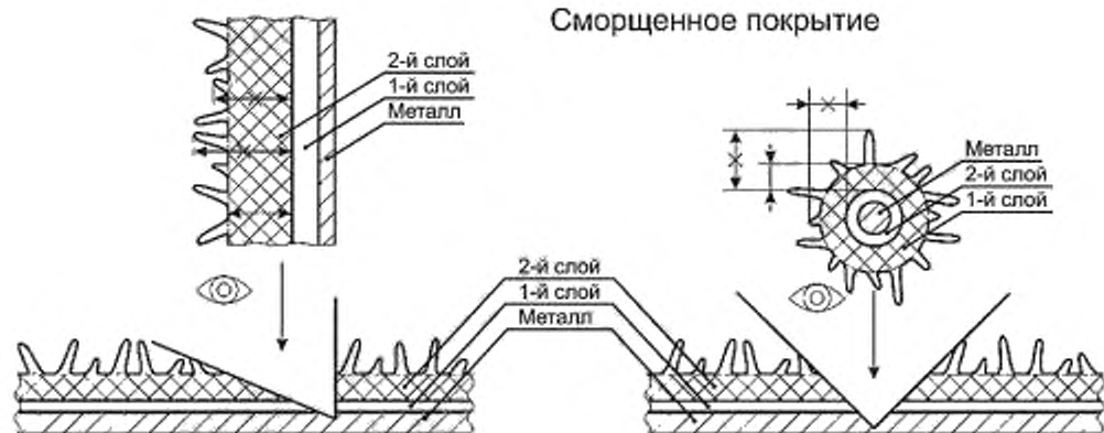
Рисунок М.1 — Внешний вид разреза покрытия при измерении толщины покрытия методом клиновидного реза
